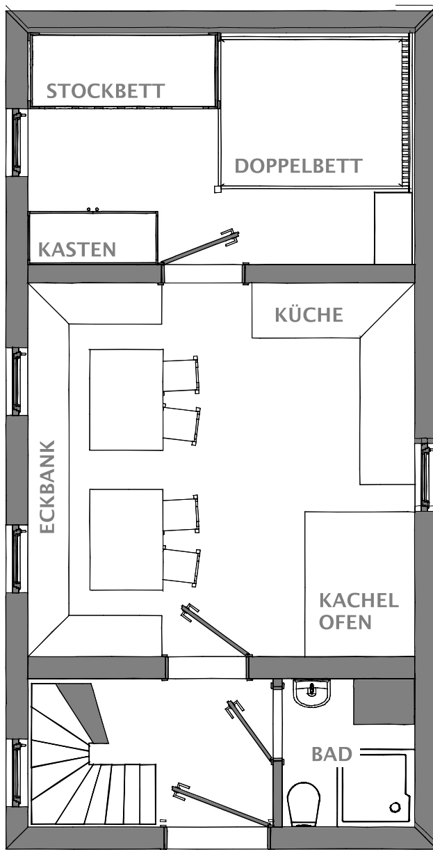
ERDGESCHOSS
