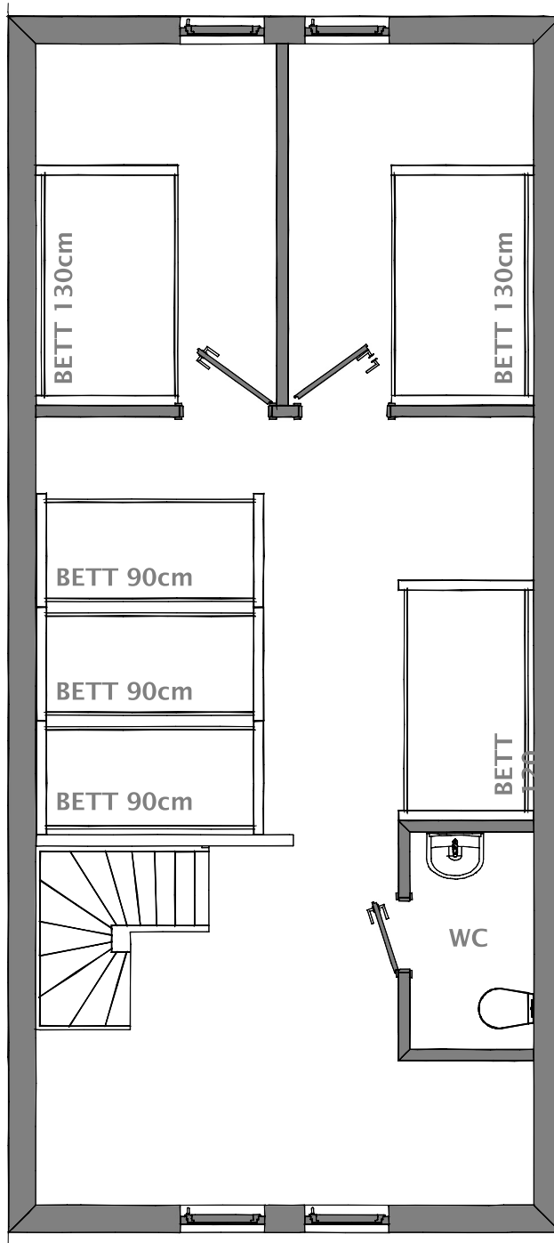
OBERGESCHOSS
